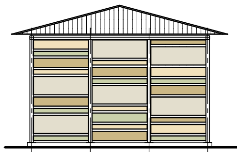
ELEWACJA BOCZNA
